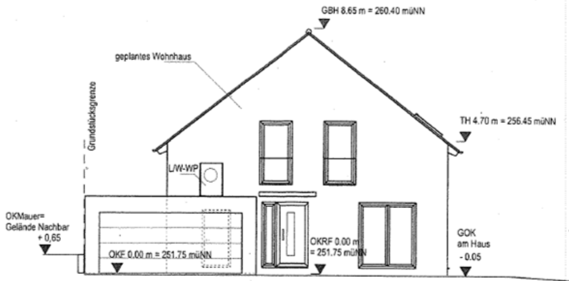
Ansicht WESTEN
